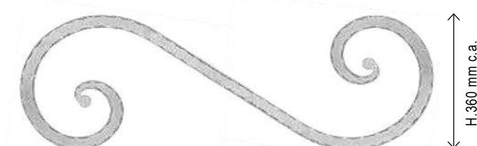
Destro / Right Martellato / Hammered H. 360 x L. 1500 mm. Art.15.157.225 \neq 30 x 8 mm
