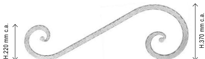
Sinistro / Left Martellato / Hammered H. 370 x L. 1500 mm. Art.15.157.200 \neq 30 x 8 mm
