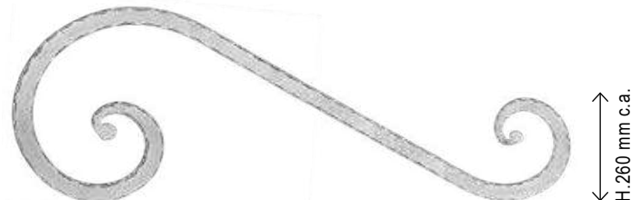
Destro / Right Martellato / Hammered H. 460 x L. 1500 mm. Art.15.157.210 \neq 30 x 8 mm
