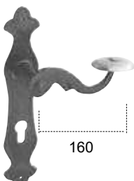
H. 230 X L. 50 mm. Art. 16.021 (a coppia)
